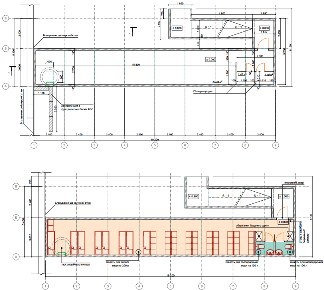
Рис. 1. Кресленник модульного укриття
