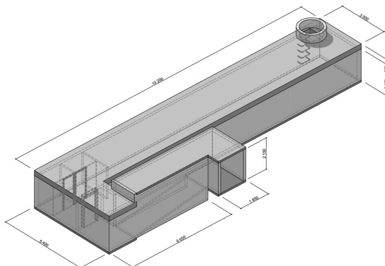
Рис. 2. Загальний вигляд конструкції ПРУ 6
